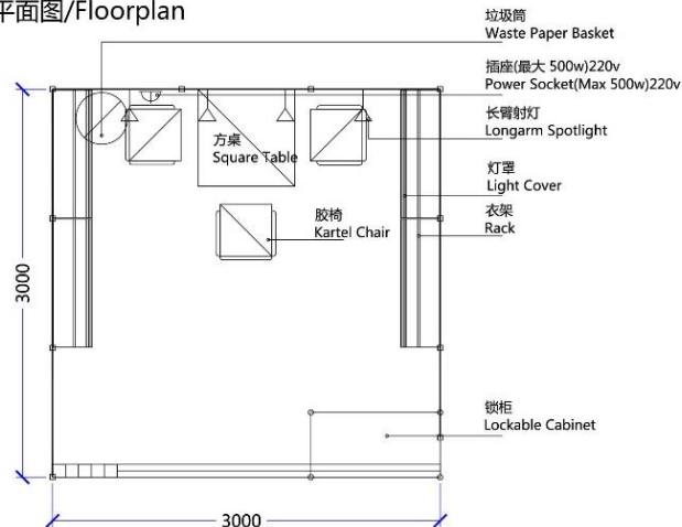
平面图/Floorplan
