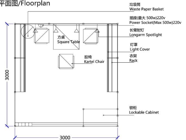
平面图/Floorplan
